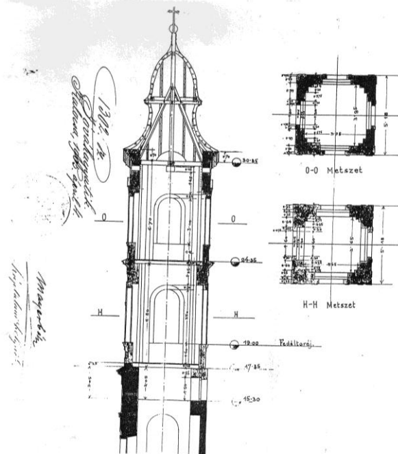
Az újonnan építendő torony tervrajza az Érseki Hatóság jóváhagyásával (A számadatokból leolvasható, hogy kb. 40 m magas)
