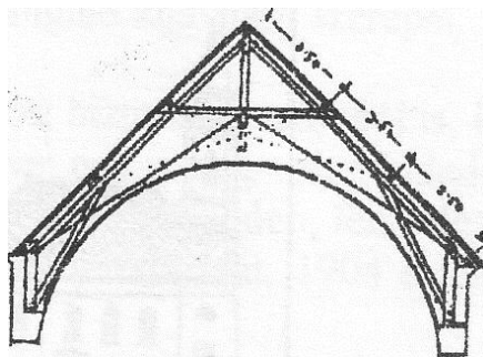
Az Ardand fedélszék Petrovác-féle változata
