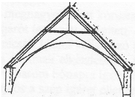
Wiegmann fedélszék
